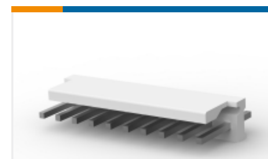
TE Part # 1-644752-0 10P MTA156 HDR ASSY SQ STR F/L
